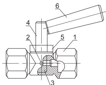
Рис. 11. Устройство 3-х ходового крана
