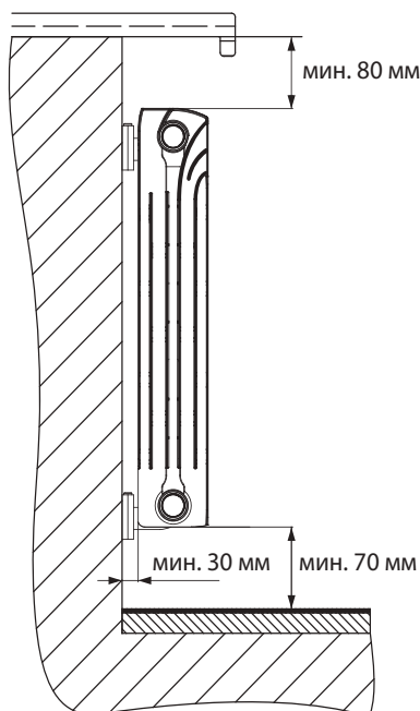
Рис. 18. Правила установки радиаторов STOUT Space и Space Ventil
