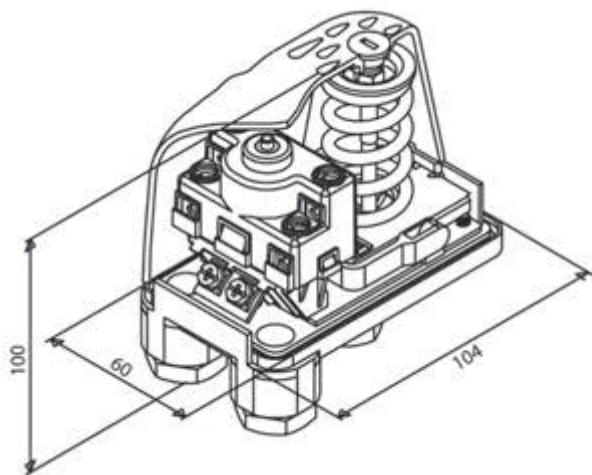
Рис. 27. Габаритные размеры реле «сухого хода»
