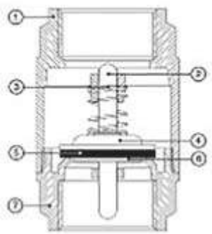
Рис. 33 Устройство обратного клапана с пластиковым затвором
