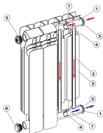
Рис. 14. Устройство радиаторов STOUT Space и Space Ventil.
