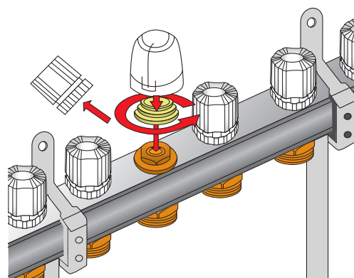
Рис. 12. Установка термoeлектропривода
