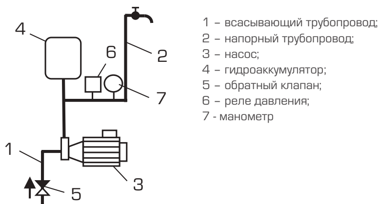
Рис. 20. Схема водоподъемной установки системы водоснабжения
