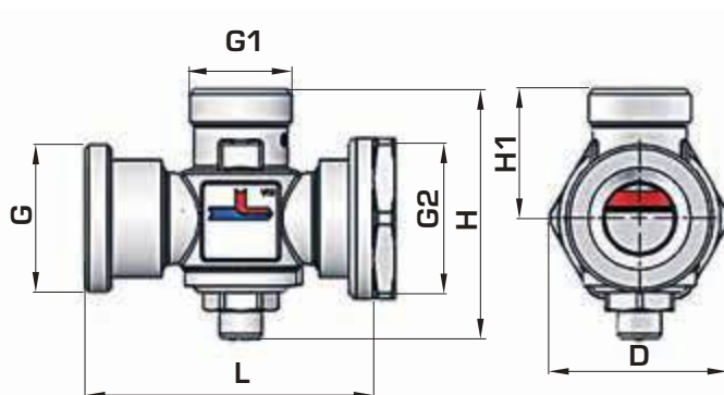
С внутренней резьбой
