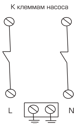
Рис. 29. Схема электрических соединений реле «сухого хода»
