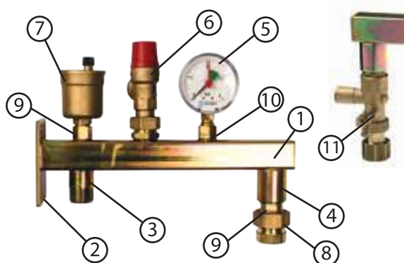
Рис. 17. Устройство группы безопасности для расширительных баков
