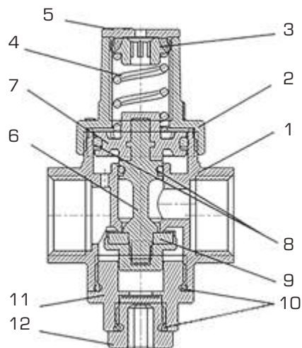
Рис. 15. Устройство редуктора SVS-1009 (1010)
