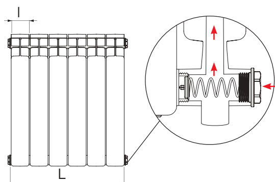
Рис. 5. Устройства перераспределения потока теплоносителя через секции радиатора Bravo
