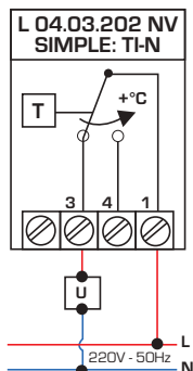
Рис. 4. Схема электрических соединений
