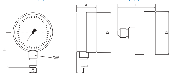
Радиальное присоединение штуцера
