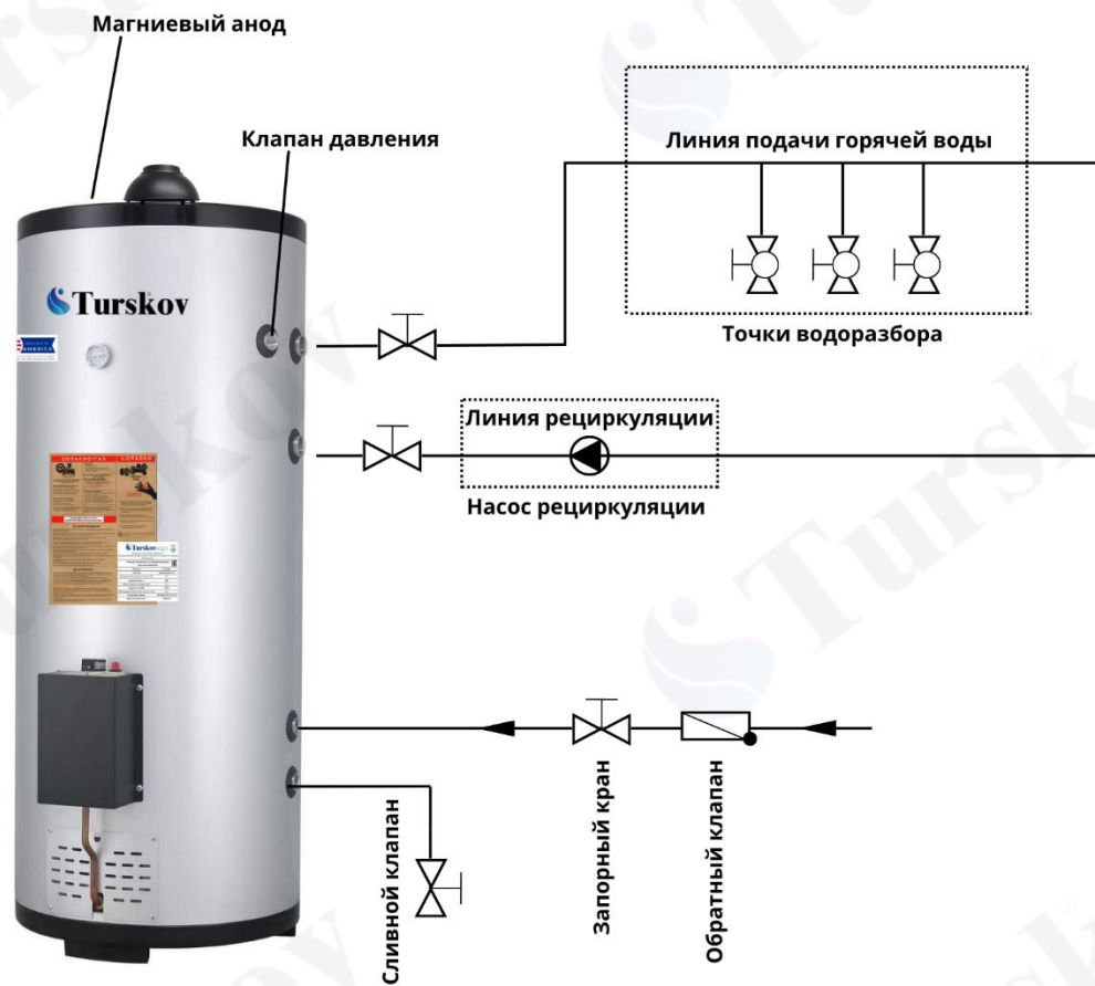
Схема 2. Подключение к сети водоснабжения.
